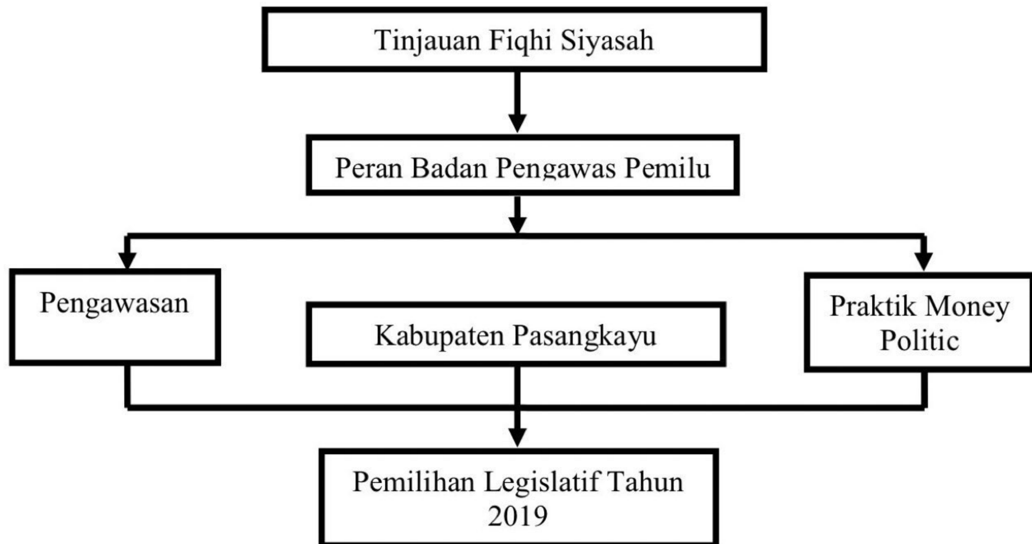
Gambar 2.1 Kerangka Pemikiran
